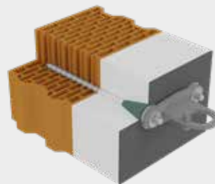
Montage Hohllochziegel auf Vollwärmeschutz
